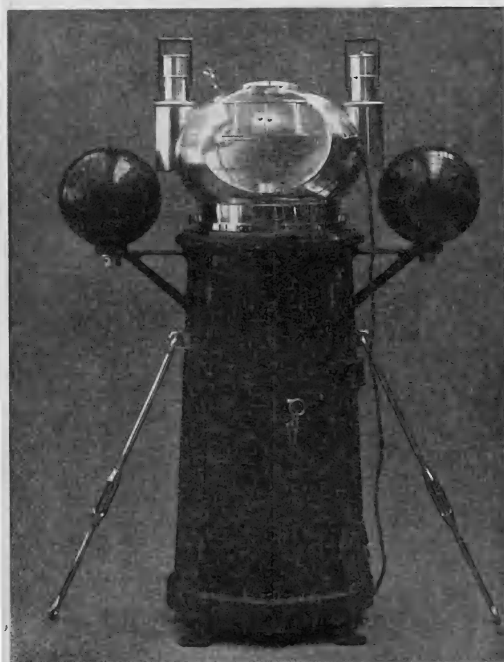
2. Закрытый судовой компасъ въ колпакѣ съ нактоузомъ, крѣпленіемъ и желѣзными шарами для уничтоженія девиціи.
